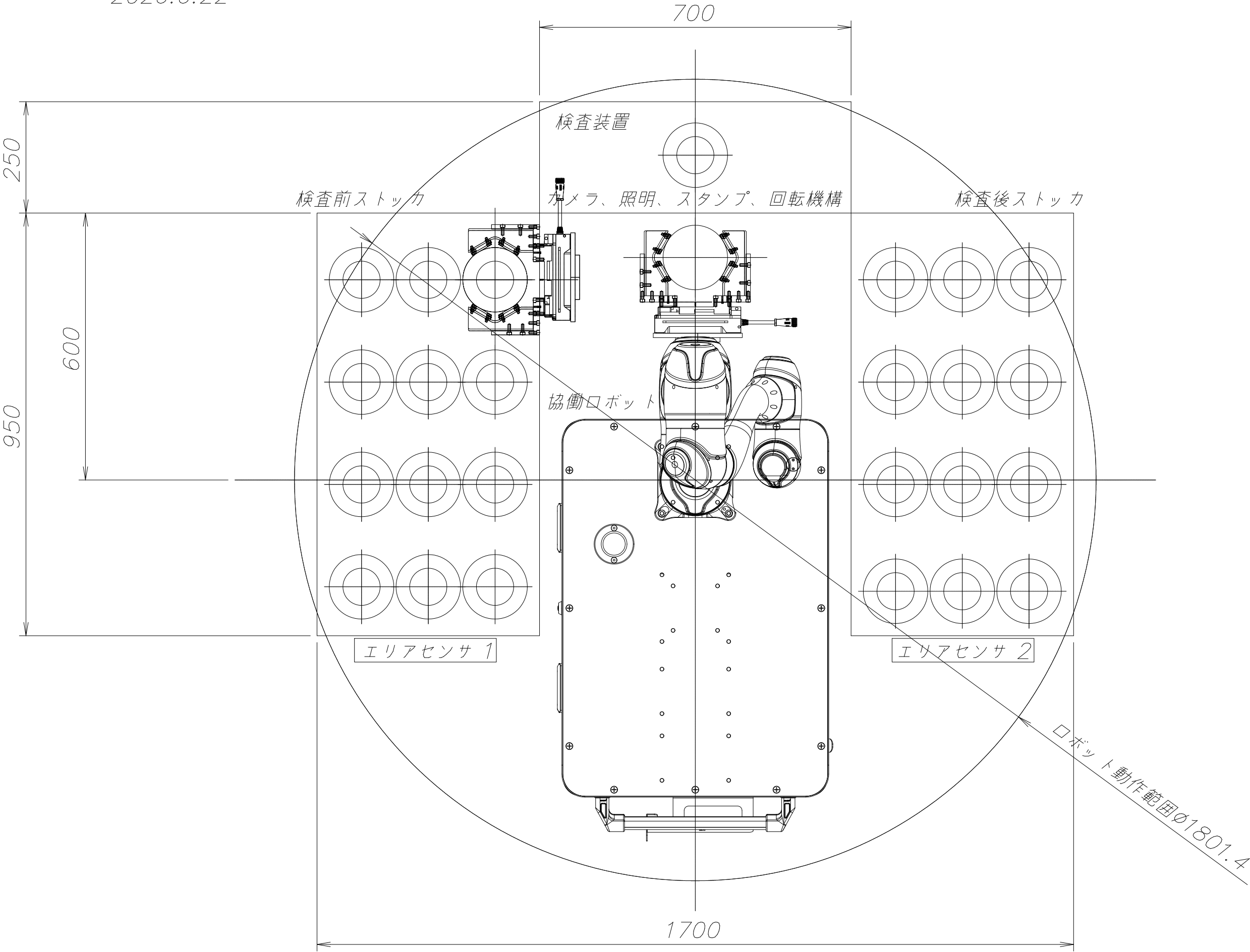
外観検査装置 全体レイアウト図 2026.6.22
